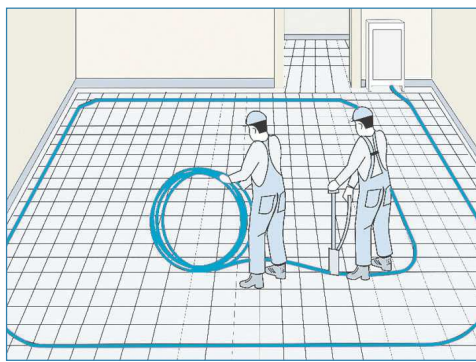
Подающую часть трубы подсоединить к коллекторной группе, укладывать с требуемой плотностью (с удвоенным шагом), шпильками крепить трубы в соответствующих местах.
