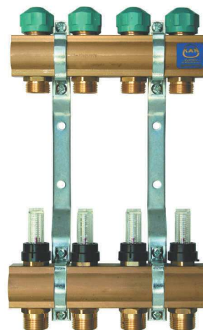
коллекторная группа серии 75A
